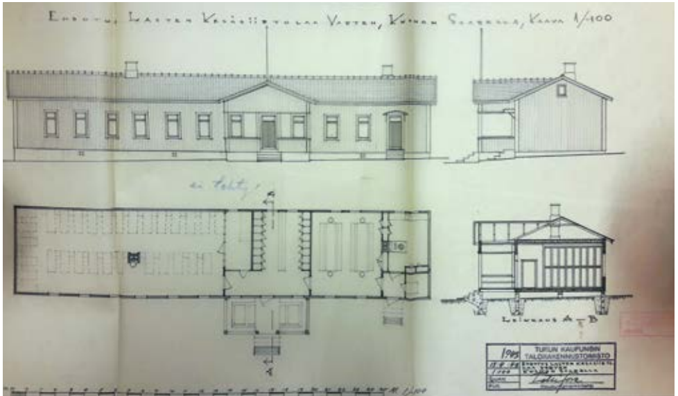
Totti Soran mallipiirustus vuodelta 1941. Tilapalvelukeskus, kuva KK.
