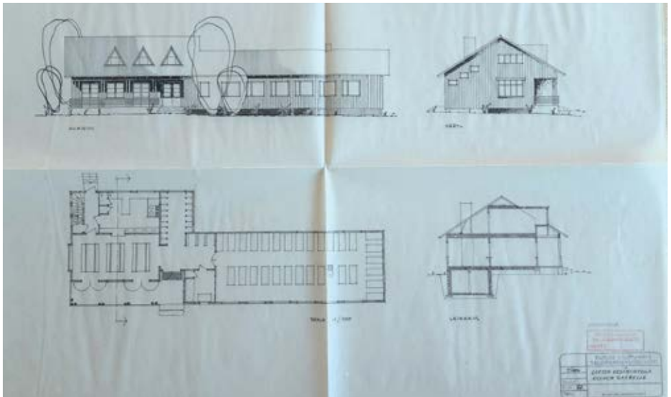
Hiekkapohjan pohjapiirustus. Turun kaupungin Talorakennusosasto, Arne Ehojoki 1949.
